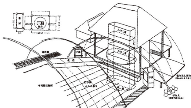
上三原田の歌舞伎舞台 機構図
